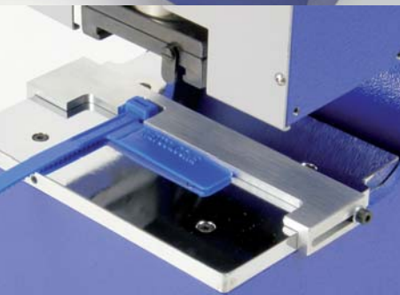
Typenhalter mit Schnellwechsellvorrichtung (SV)
